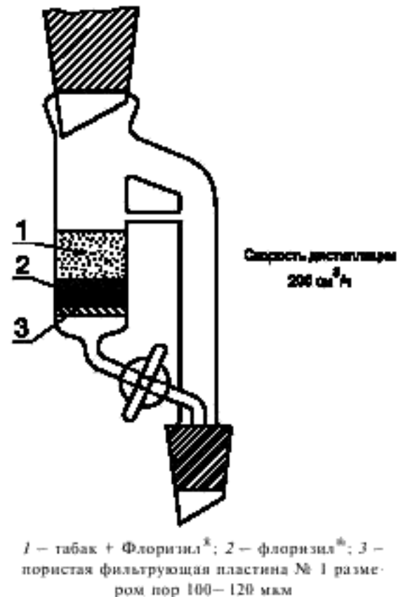
Рисунок 1 — Часть аппарата Сокслета, используемая для экстракции табака
