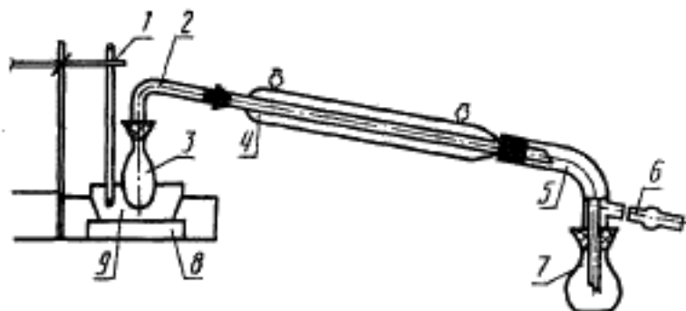
1—термометр; 2—соединительная трубка; 3—грушевидная колба вместимостью 75 мл; 4—холодильник Либиха; 5—аллонж; 6—хлоркальциевая трубка; 7—колба-приемник; 8—закрытая плитка; 9—баня со сплавом Вуда
